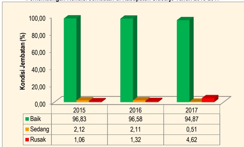
Perkembangan Kondisi Jembatan di Kabupaten Sidoarjo Tahun 2015-2017
