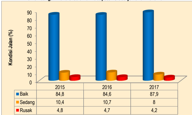
Perkembangan Kondisi Jalan di Kabupaten Sidoarjo Tahun 2015-2017
